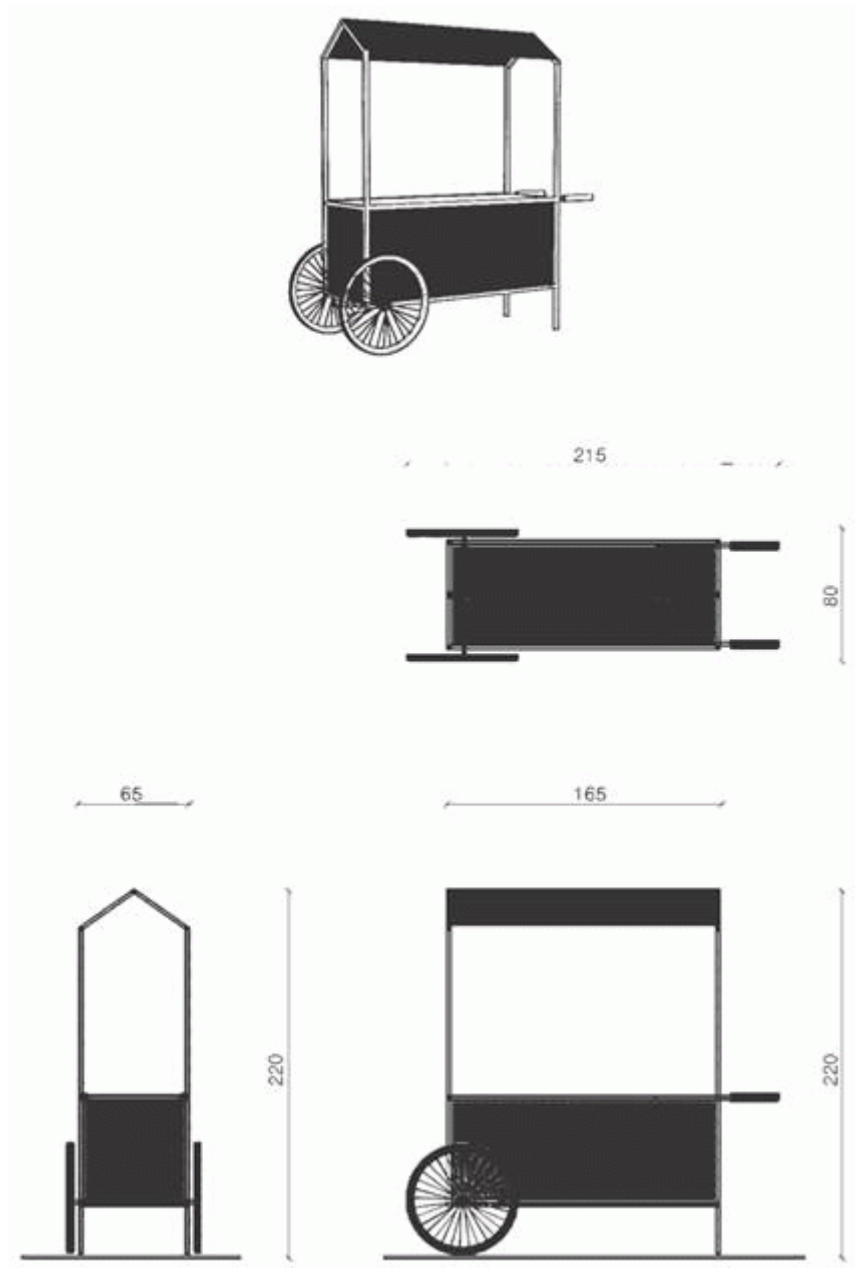
Grafički prilog br. 3: Mobilna tezga "MT 2015"
