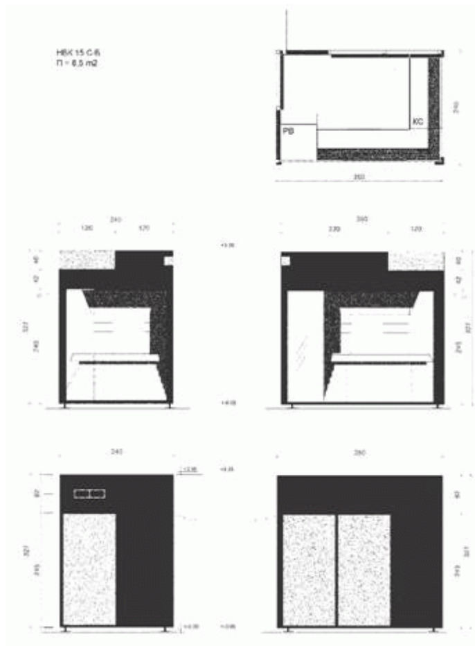
Grafički prilog br. 2 - Kiosk "NBK 15 S-B"
